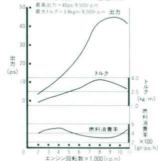
ヤマハTZR250エンジン性能曲線
